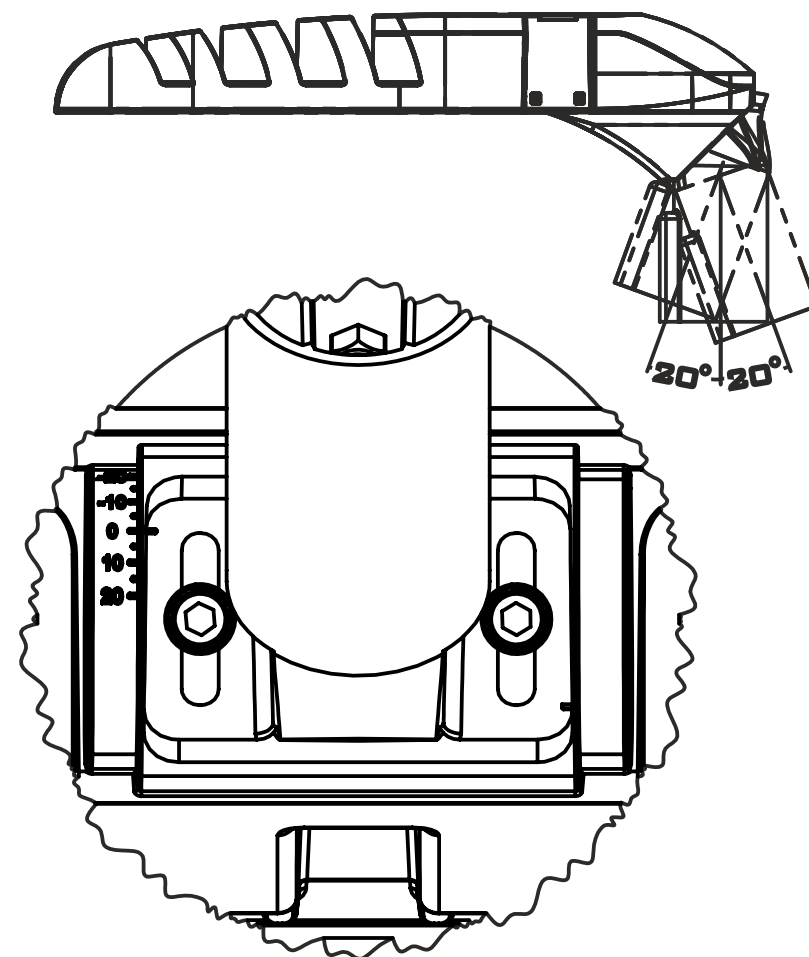
Положение кронштейна №2
