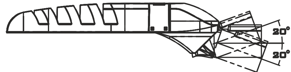
Положение кронштейна №1
